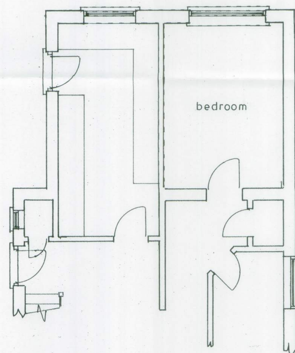
Plan 1:50
