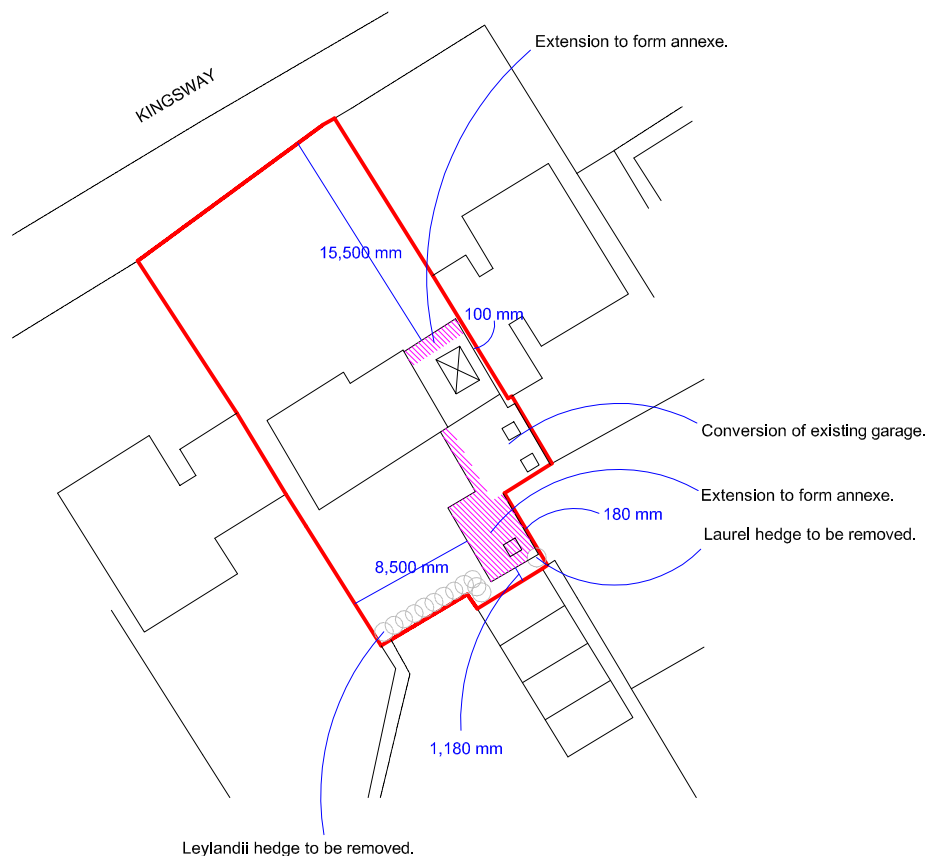
SITE PLAN - 1/500
