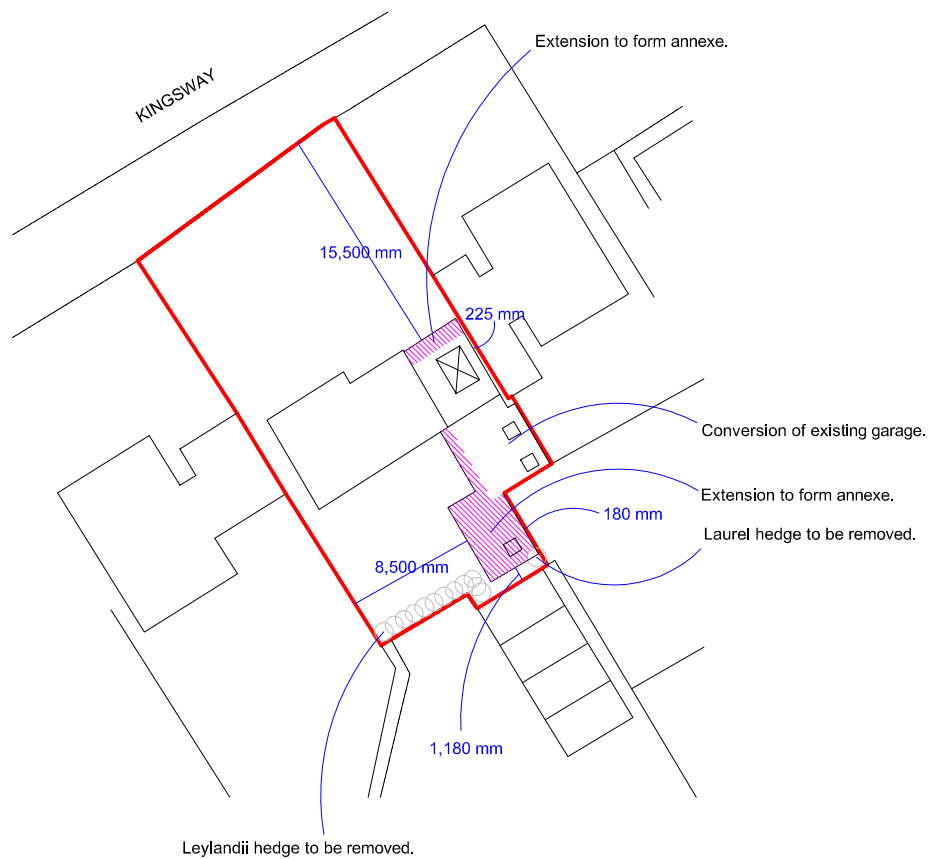
SITE PLAN - 1/500
