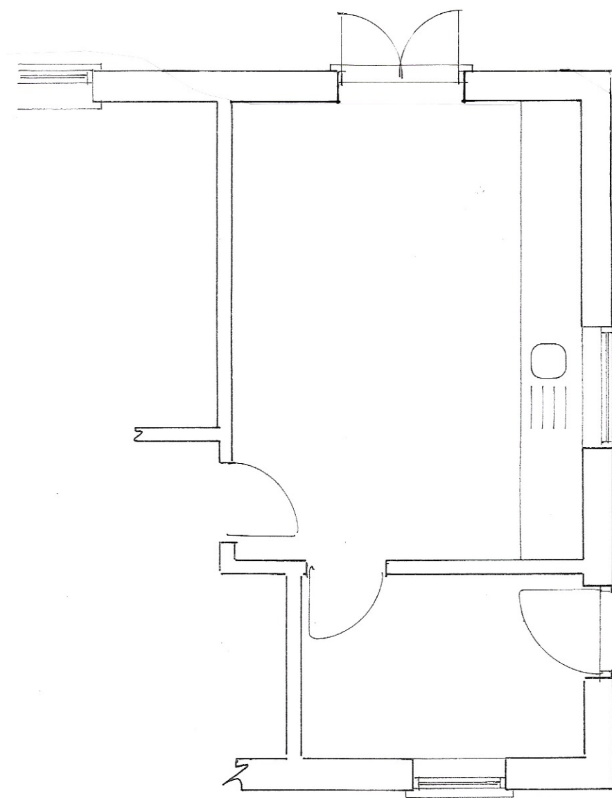
Plan 1 : 50
