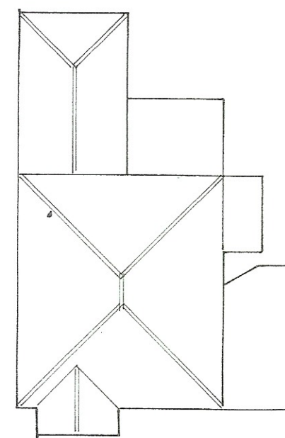
roof plan 1 : 200
