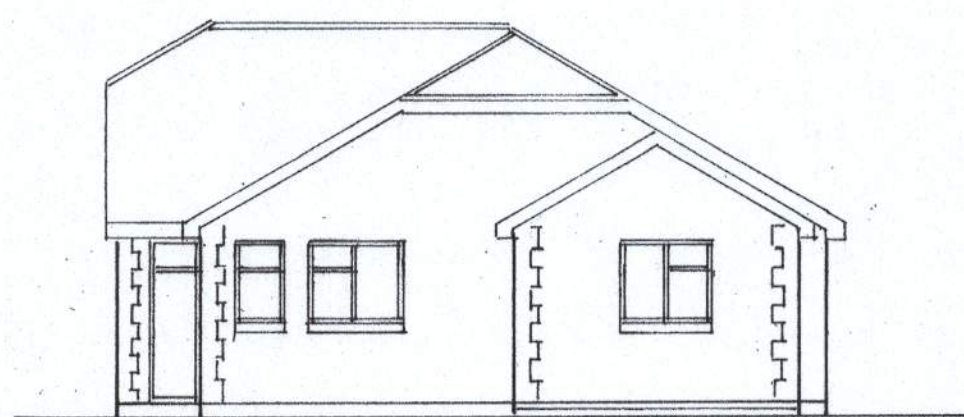
east 1 : 100
