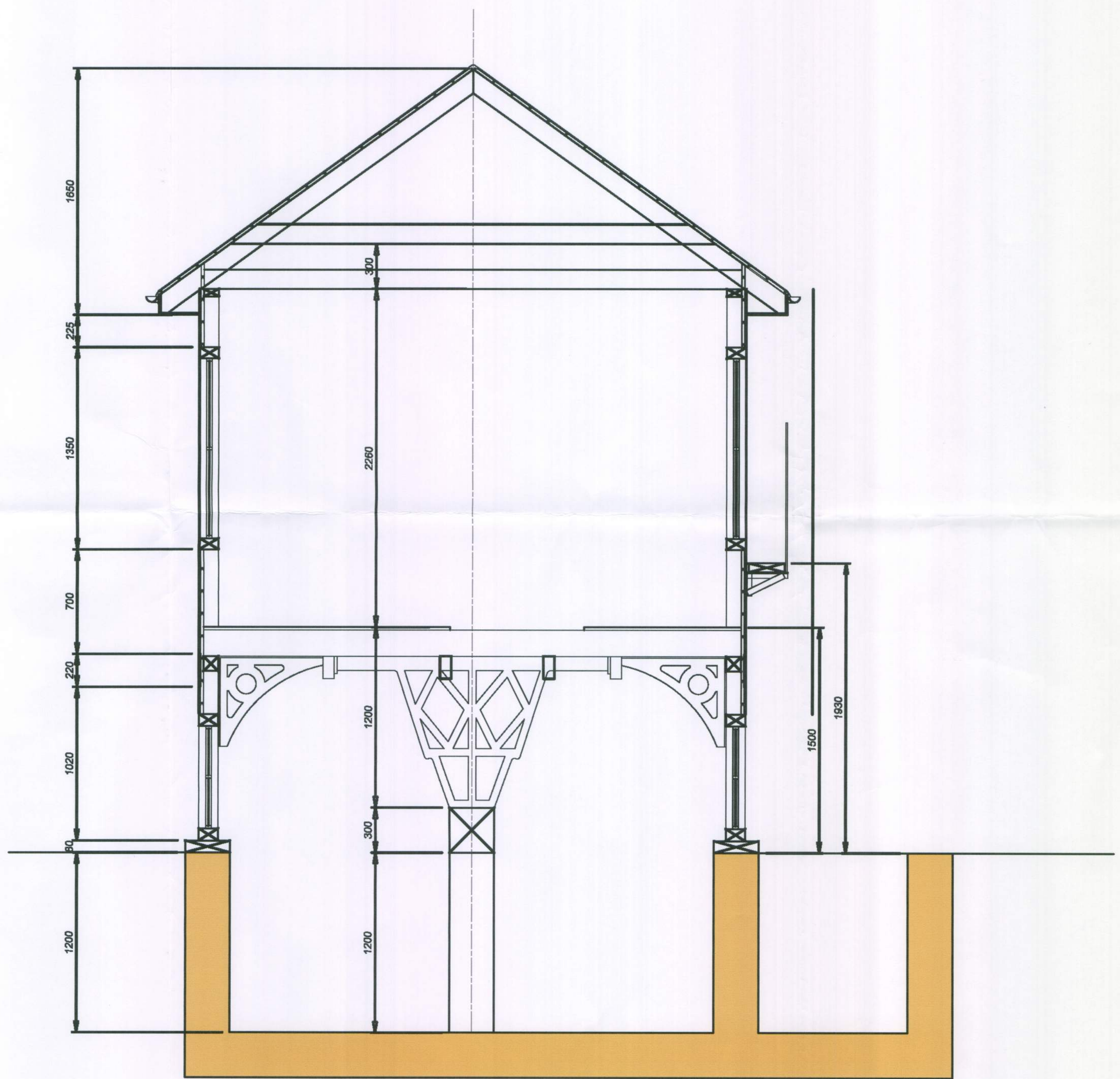
SECTION A-A scale 1:20
