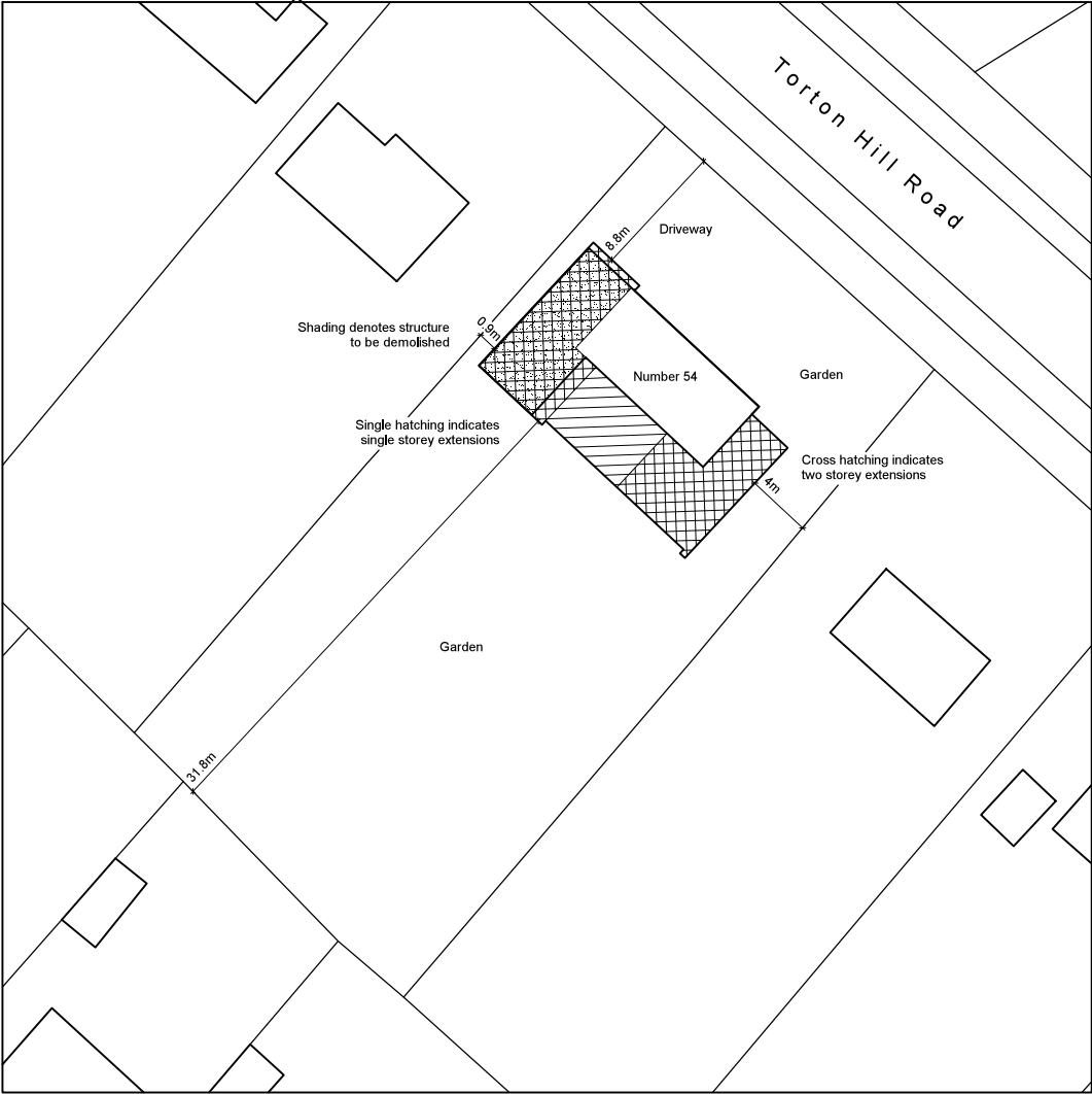
B l o c k P l a n S c a l e 1 : 5 0 0
