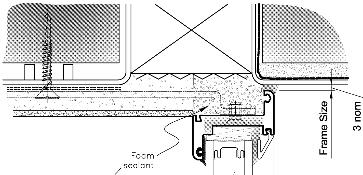
Fixing Lug
