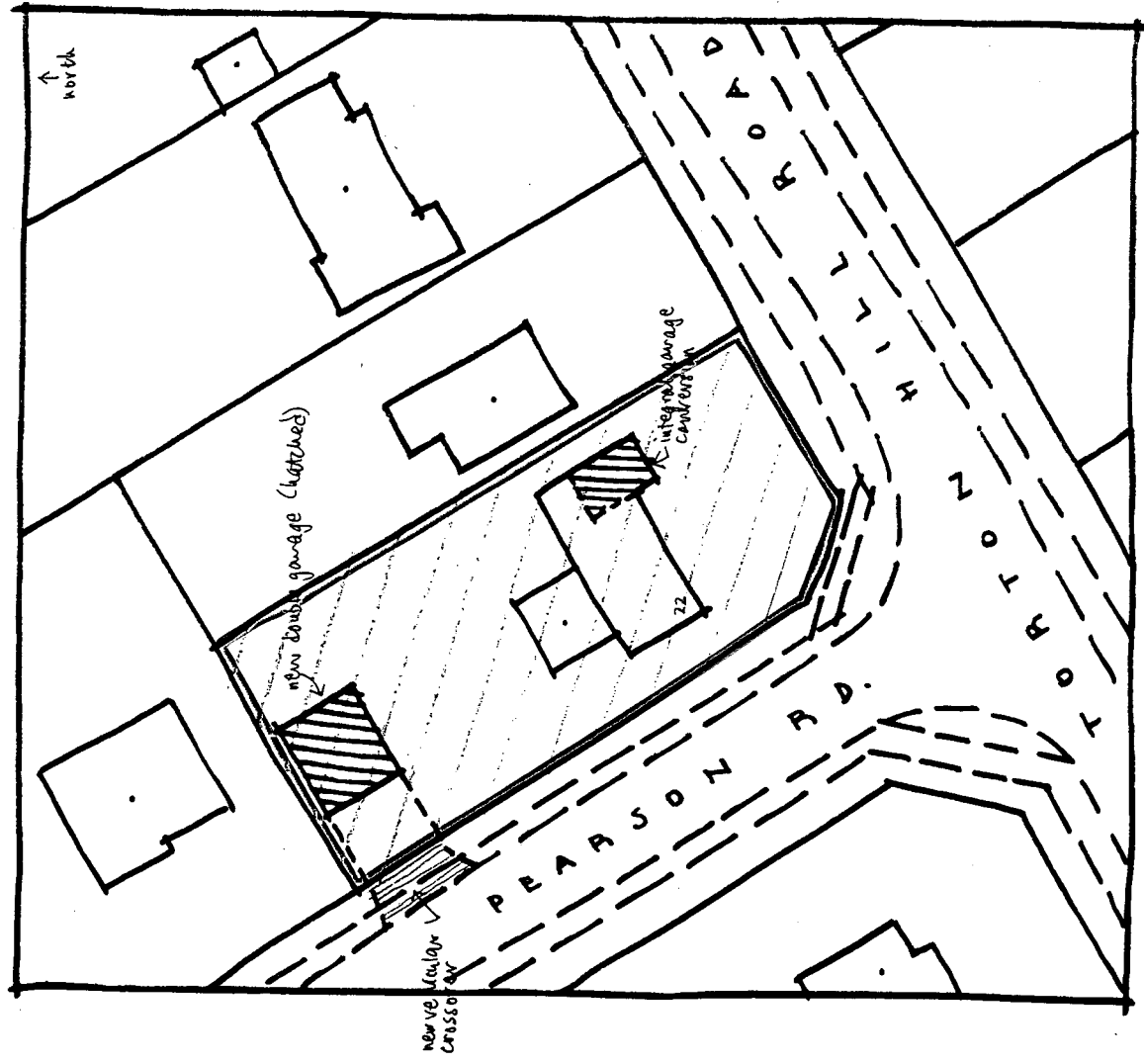
Site Plan 1:500
